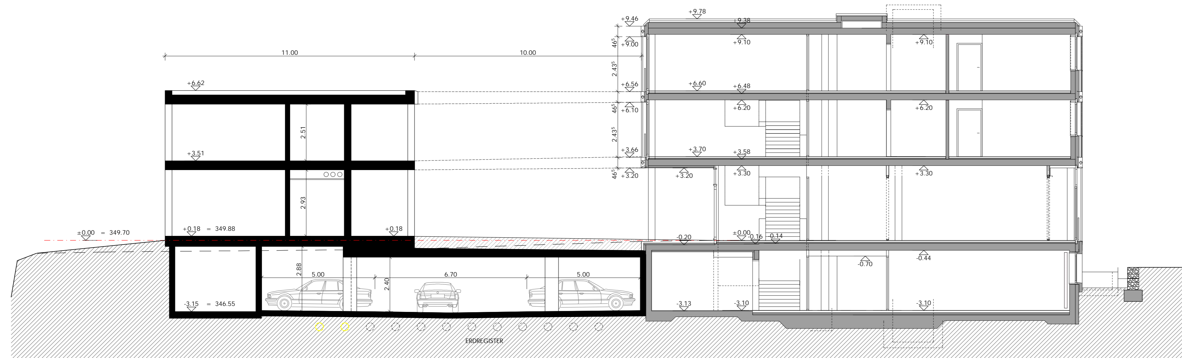
QUERSCHNITT
